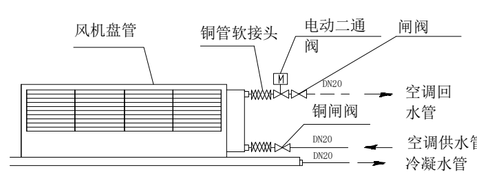
风机盘管接管示意图
